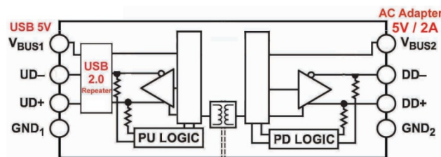
URP-301-I Self Power-5V-2A
