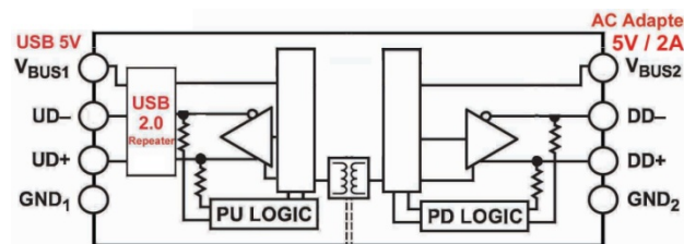
URP-401-I Self Power-5V-2A
