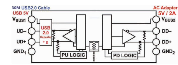
URP-301-I Self Power-5V-2A
