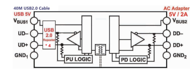
URP-401-I Self Power-5V-2A
